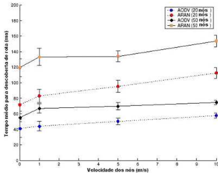
Figura 2.6: Tempo médio para Descoberta de rota
