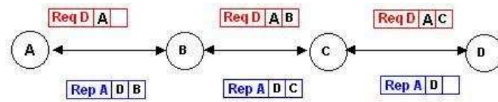
Figura 2.2: Processo de descoberta de rota - Primeiro estágio
