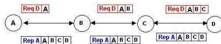
Figura 2.3: Processo de descoberta de rota - Segundo estágio
