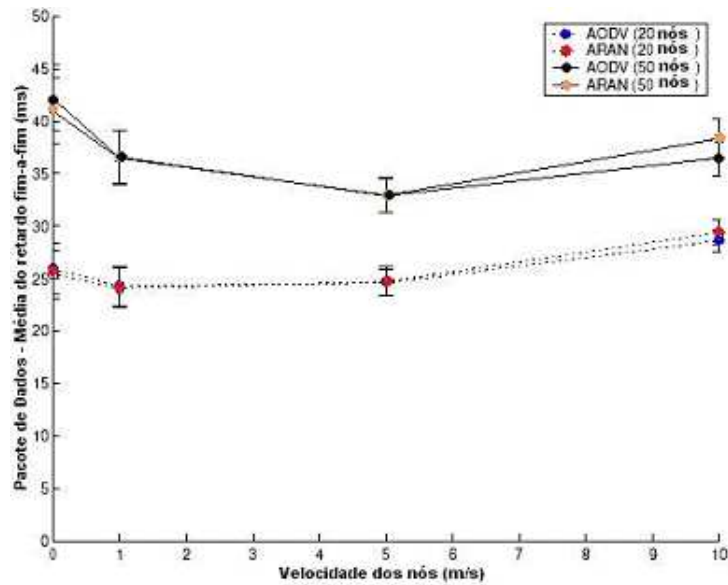
Figura 2.5: Retardo fim-a-fim para os pacotes de dados
